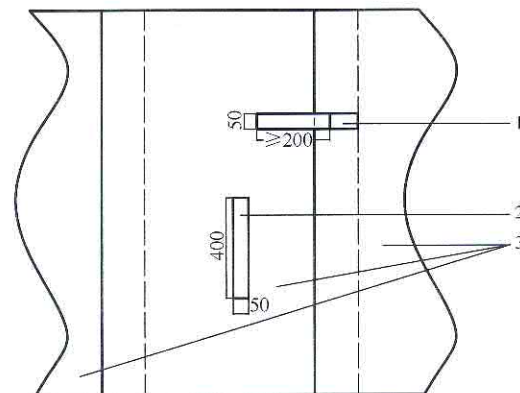
图 9.0.4 剥离强度试件
