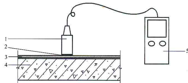
图 8.2.2 超声波法检测示意图
