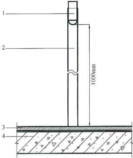
图 10.0.6 落锤法检测水平面防水层柔性示意图 1—落锤；2—导管；3—防水层；4—基层
