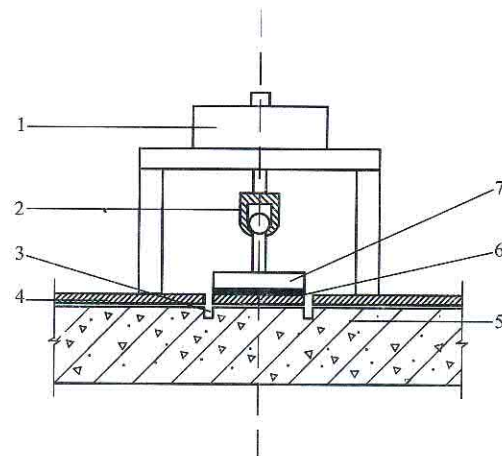
图 7.0.5 防水层粘结强度检测示意图
