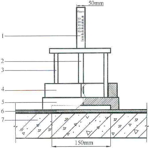
图 11.0.2 渗水仪示意图
