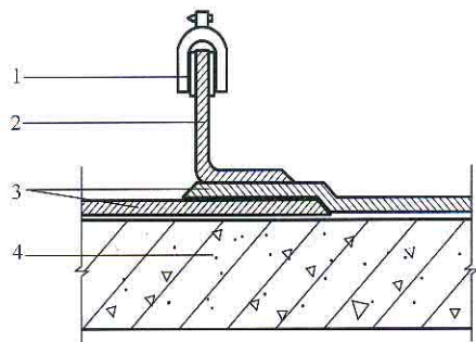
图 9.0.6-2 卷材防水层接缝剥离 强度检测示意图
