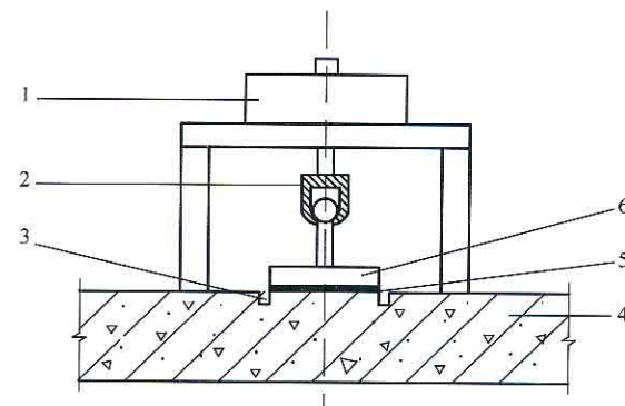
图 6.0.4 基层表面正拉粘结强度检测示意图
